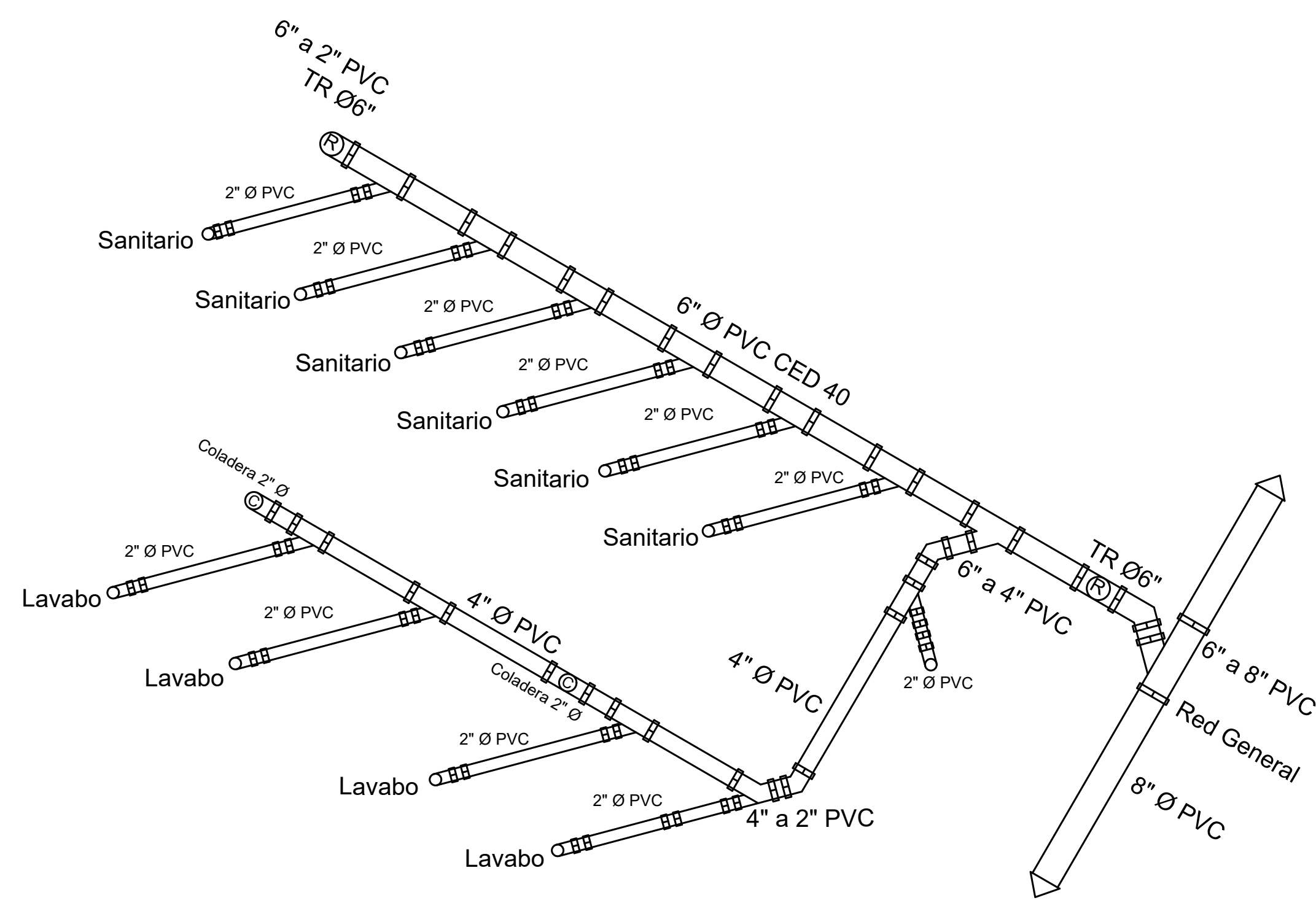
Modulo 2 (Baño de Mujeres, Taquilla y Bodega) Isometrico Instalacion Sanitaria
