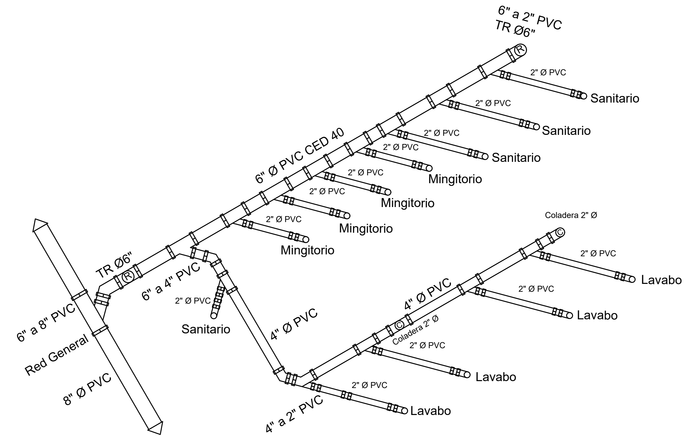
Modulo 1 (Baño de Hombre, Taquilla y Bodega) Isometrico Instalacion Sanitaria
