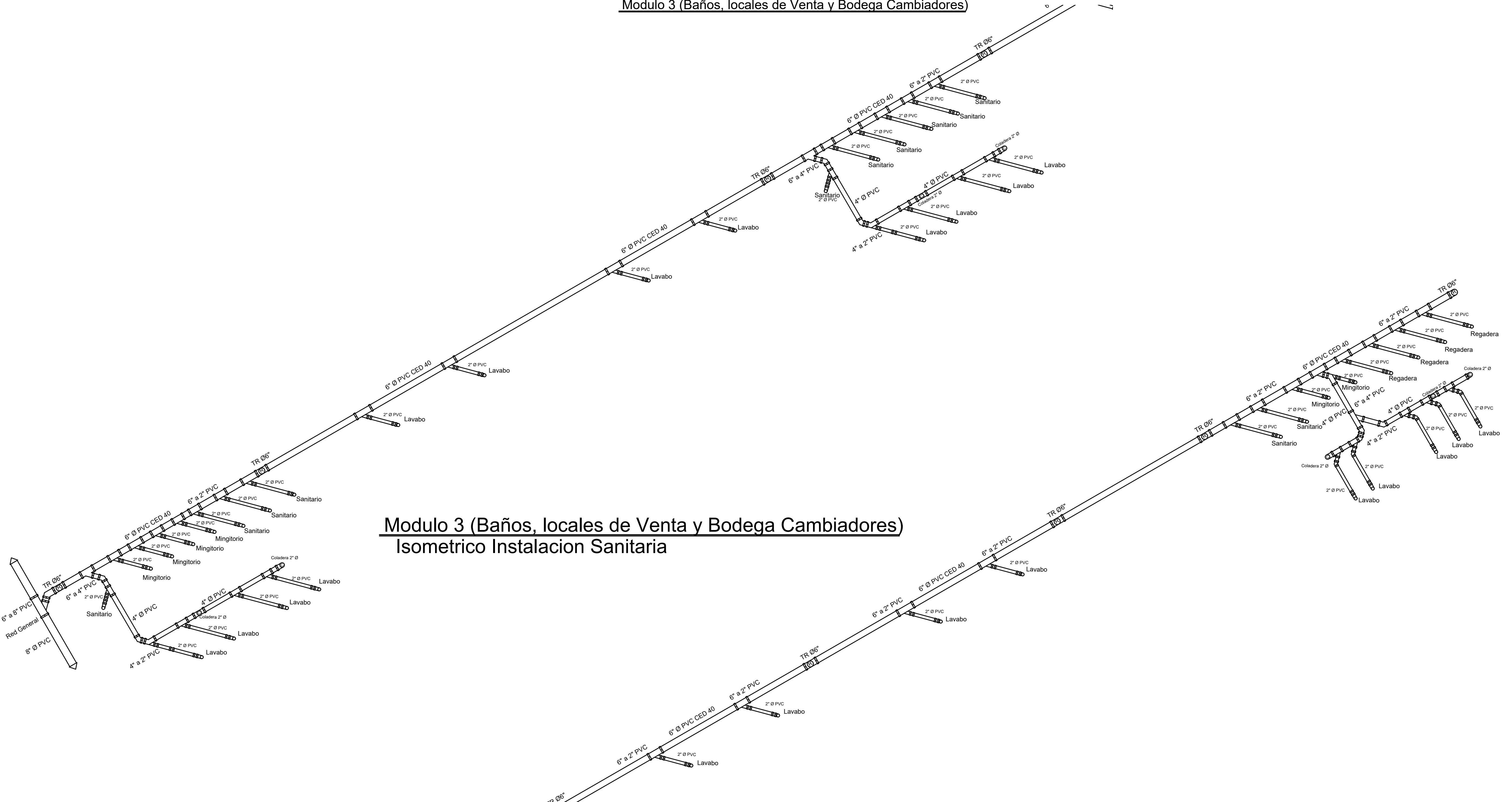
Modulo 3 (Baños, locales de Venta y Bodega Cambiadores)
